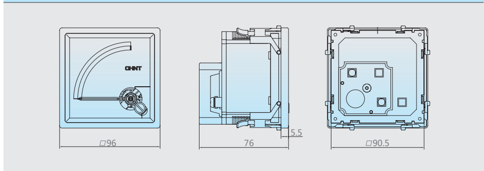
51S666 外形尺寸图
